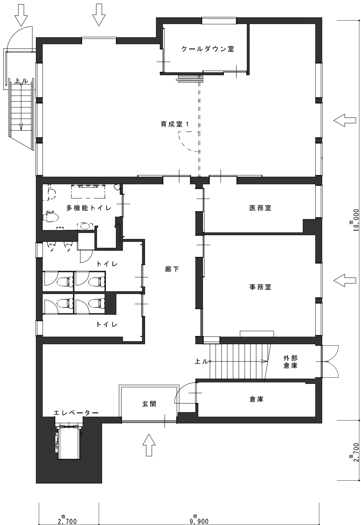
1 階 平 面 図 1 / 1 0 0
