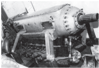
スミソニアン博物館にある 正田製「試飛六」エンジン
