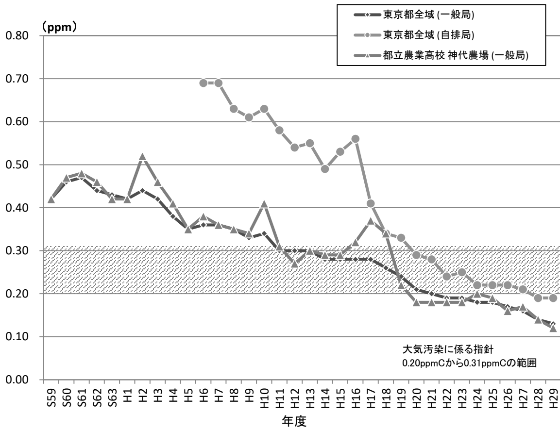
資料：東京都環境局 ※平成30年度分データの東京都データは作成時未公表 図 4-1-17 非メタン炭化水素の長期推移 (6~9時の年平均値)
