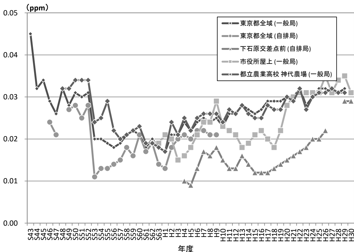
資料：東京都環境局，環境政策課 ※平成 30 年度分データの東京都データは作成時未公表 図 4-1-13 光化学オキシダントの長期推移 (昼間の 1 時間値の年平均値)
