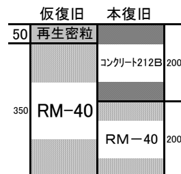
図8-2 歩道舗装(40)
