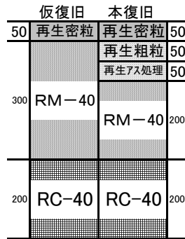
図3 高級舗装(55)
