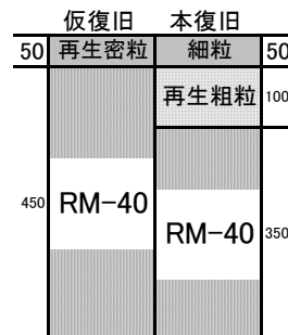
図7-3 歩道舗装(50)
