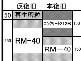
図8-1 歩道舗装(30)
