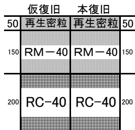
図5 簡易舗装(40)
