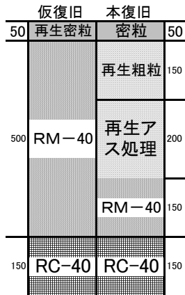
図4 中級舗装(40)
