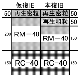
図4 中級舗装(40)
