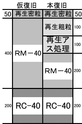
図5 簡易舗装(40)
