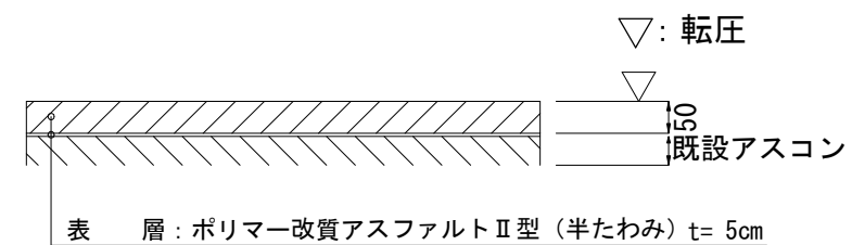
②切削オーバーレイ工 S=1:50 (1:25)
