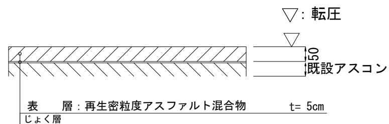
①切削オーバーレイ工 S=1:50 (1:25)
