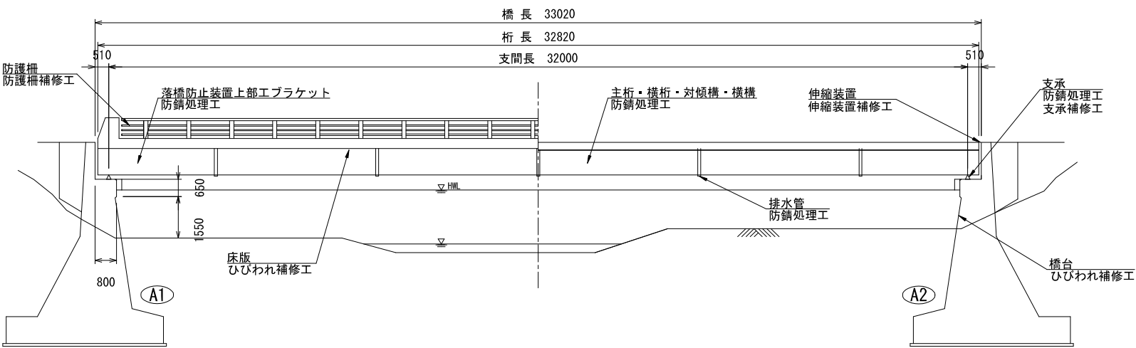
側面図 S=1/200 (1/100)
