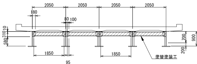
断面図 (中間横桁位置) S=1/120 (1/60)
