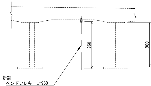
導水管設置工 詳細図 S=1/40(1/20)
