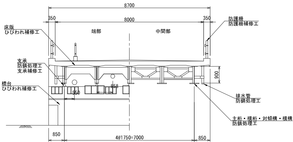
断面図 S=1/120 (1/60)
