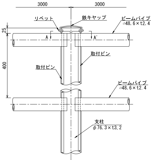
連結部詳細図 S=1/10 (1/5)
