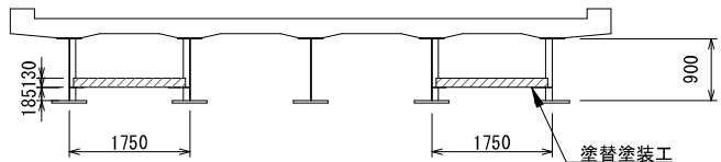
断面図 (横構位置) S=1/120 (1/60)
