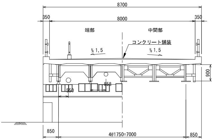
断面図 S=1/120 (1/60)
