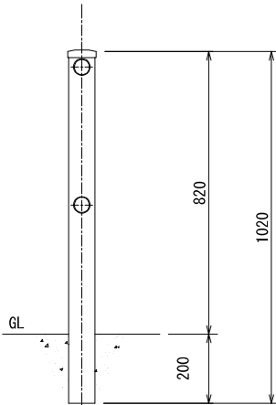
支柱設置詳細図 S=1/20 (1/10)
