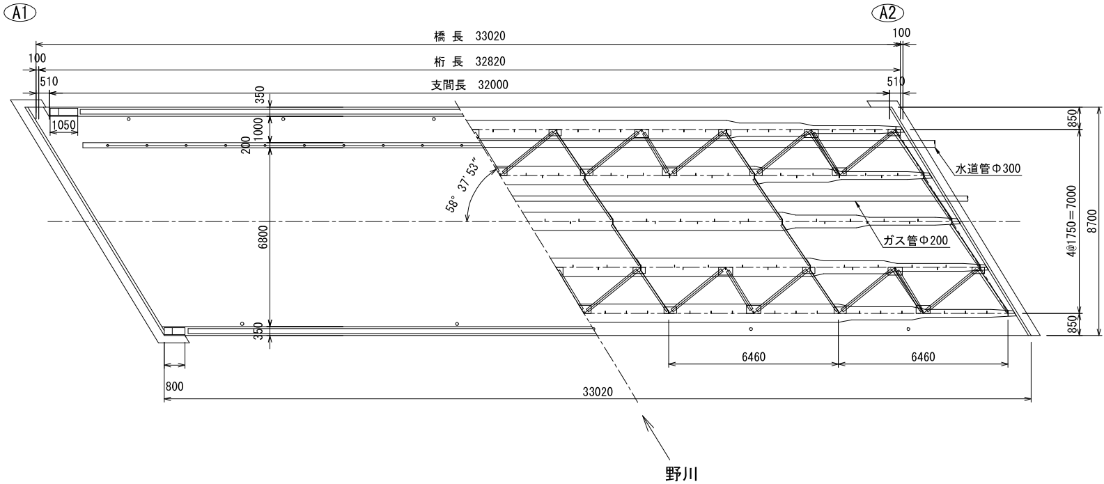
平面図 S=1/200 (1/100)
