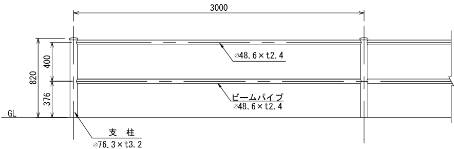
設置図 S=1/40 (1/20)
