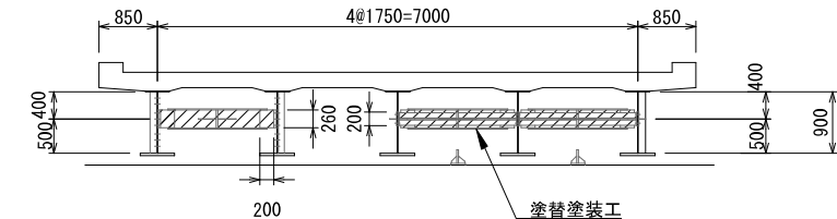
断面図 (落橋防止装置上部エブラケット位置) S=1/120 (1/60)
