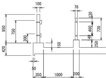
防護柵断面図 S=1/60 (1/30)
