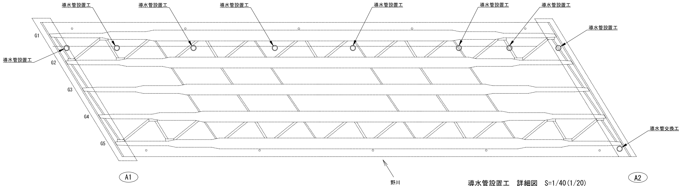
導水管設置工 詳細図 S=1/40(1/20)
