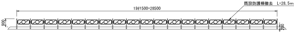
既設 横断防止柵側面図 S=1/200 (1/100)
