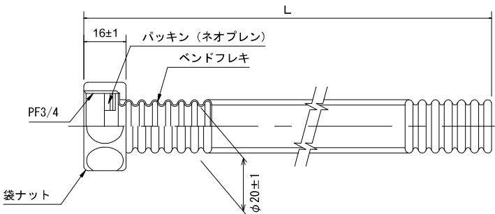
導水管詳細図 S=1/2(1/1)
