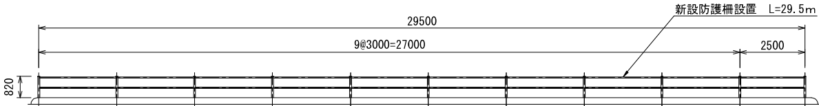
新設 横断防止柵側面図 S=1/200 (1/100)
