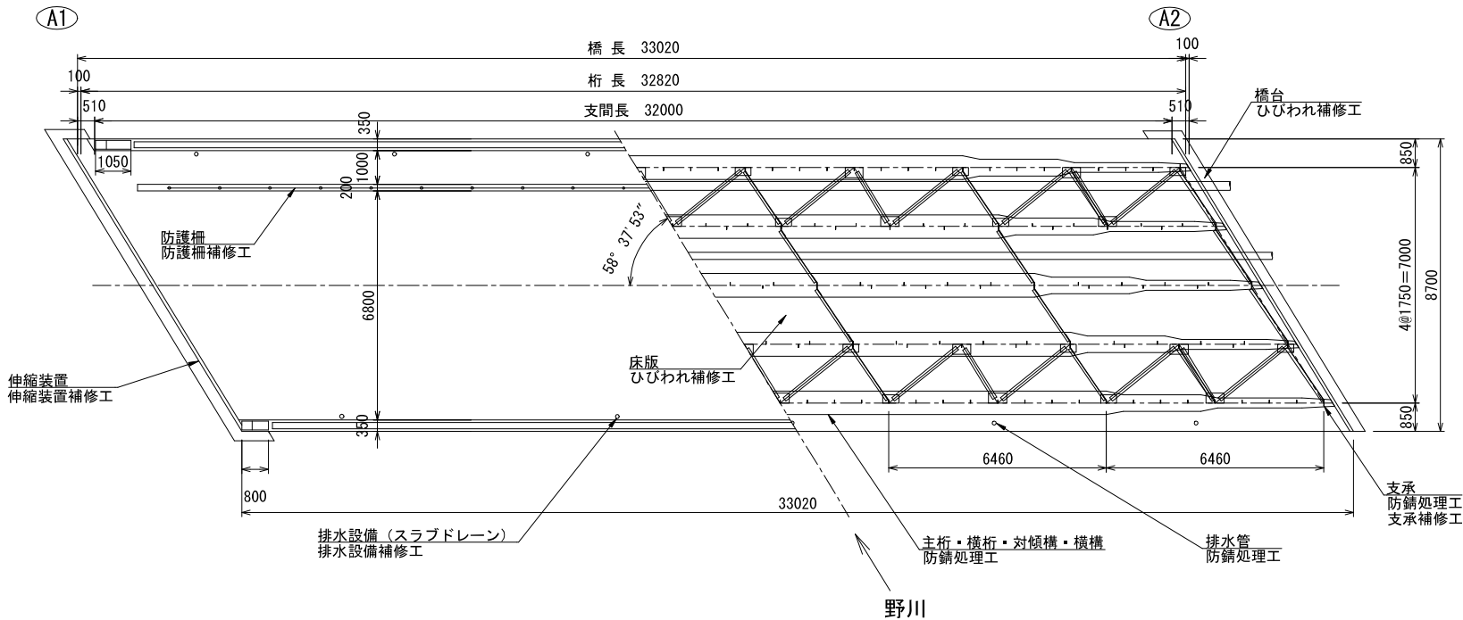
平面図 S=1/200 (1/100)
