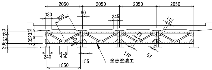
断面図 (対傾構位置) S=1/120 (1/60)
