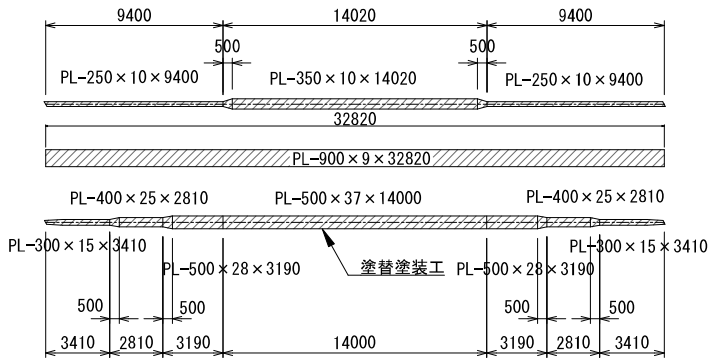
主桁詳細図 S=1/400 (1/200)
