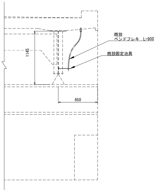
導水管交換工 詳細図 S=1/40(1/20)
