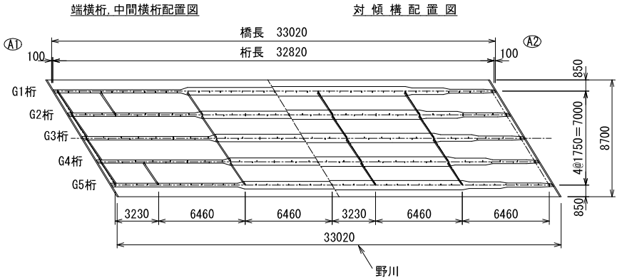
平面図 S=1/400 (1/200)
