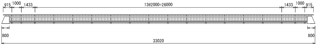
横断防止柵側面図 S=1/200 (1/100)
