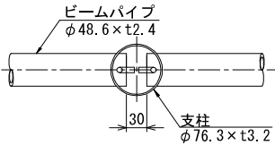
A-A' 断面図
