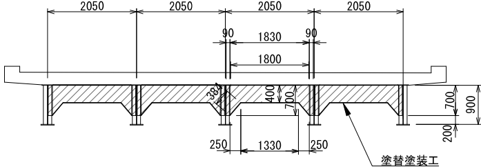
断面図 (端横桁位置) S=1/120 (1/60)
