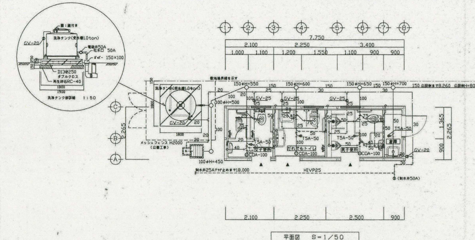
トイレ・排水電気設備図 参考図
