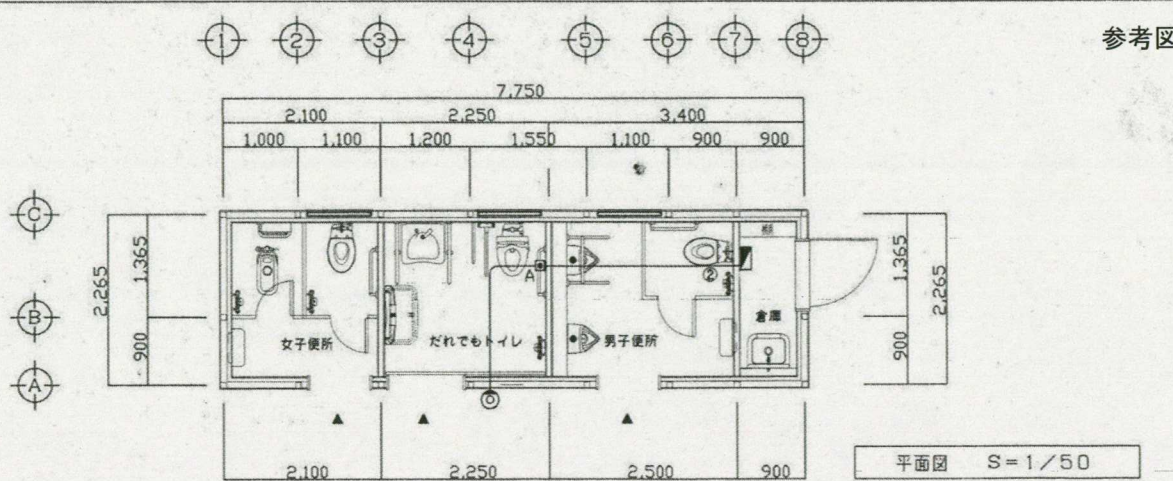
トイレ・排水電気設備図 参考図
