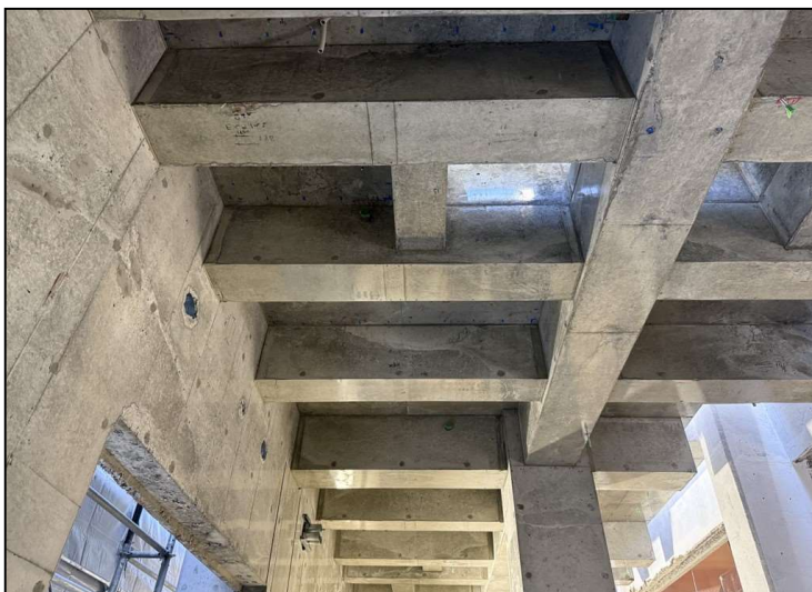
No.3 調布市立多摩川小学校給食室改修工事 増築棟躯体 施工状況
