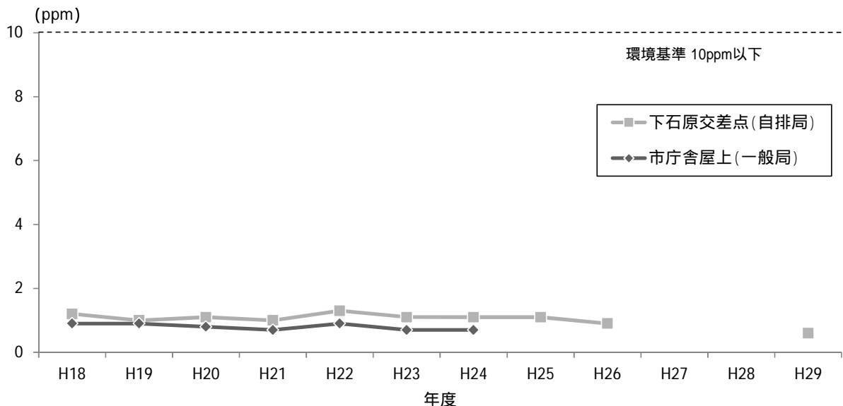
図 4-1-5 一酸化炭素の長期的評価の推移（日平均値の 2% 除外値）
