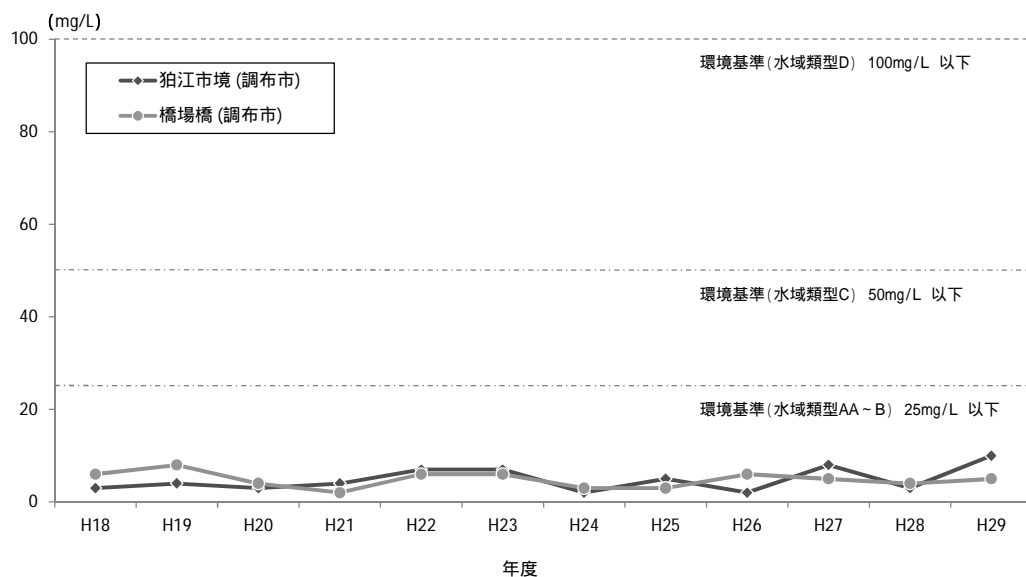
図 4-2-7 野川における浮遊物質(SS)の推移 (年平均値)
