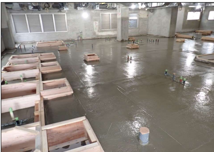
No.3 調布市立富士見台小学校給食室改修工事 内部シンダーコンクリート 施工状況
