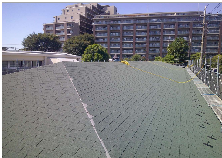
No.6 調布市立上ノ原小学校北校舎外部改修工事 屋根改修 施工状況
