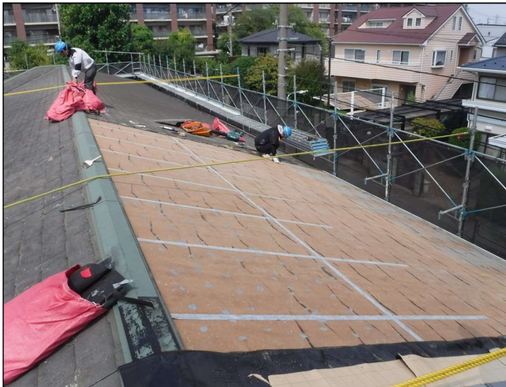
No.5 調布市立上ノ原小学校北校舎外部改修工事 屋根改修 施工状況
