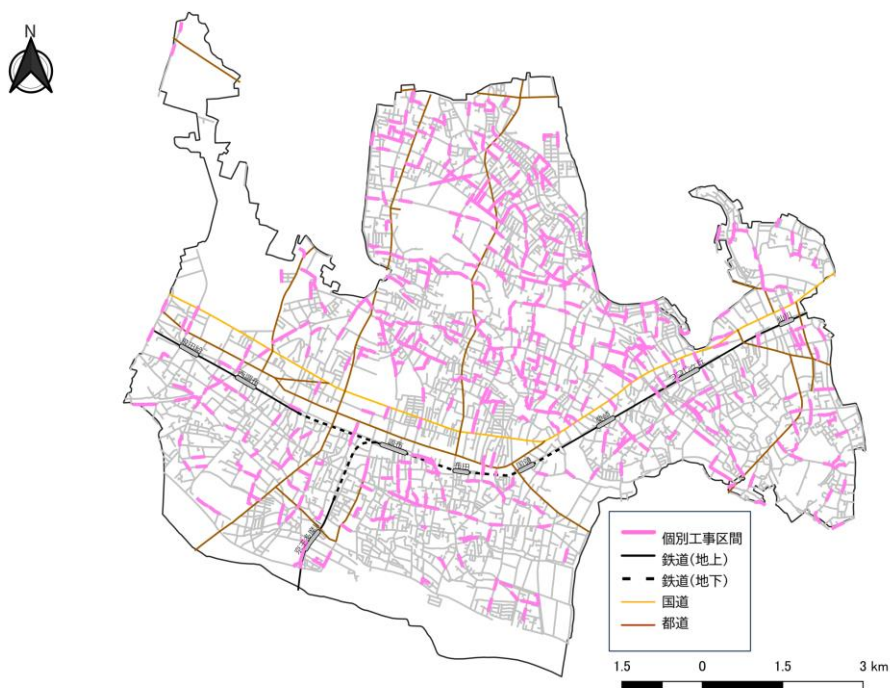
図1 短期計画対象路線図
