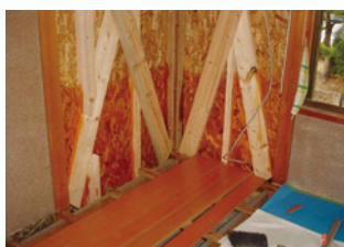
押入れ内補強
