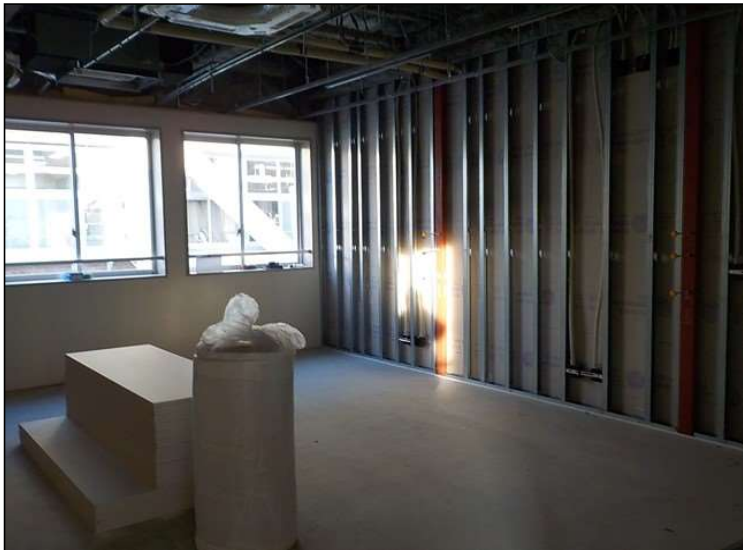
No.5 調布市立北ノ台小学校特別支援学級教室整備工事 内部改修 施工状況
