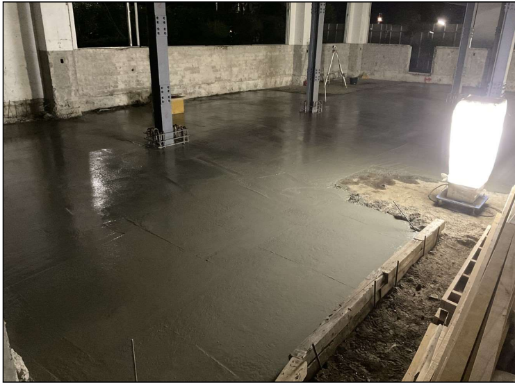
No.1 調布市立深大寺小学校給食室改修工事 床コンクリート 施工状況
